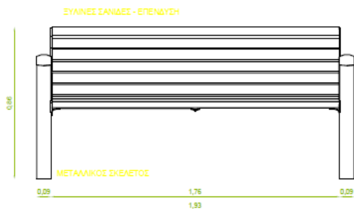
ΟΨΗ ΚΑΘΙΣΤΙΚΟΥ
