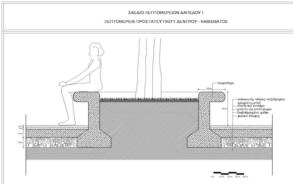
Σχέδιο 8: Κατασκευαστική λεπτομέρεια προστατευτικού δέντρου-καθίσματος
