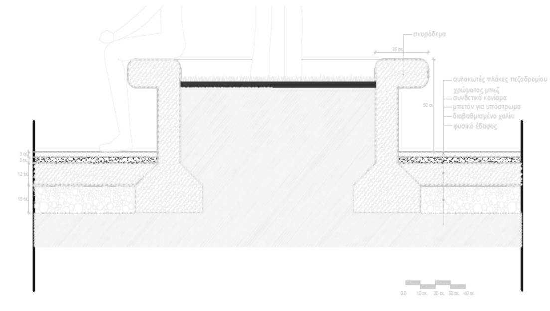
Κατασκευαστική λεπτομέρεια προστατευτικού δέντρου-καθίσματος
