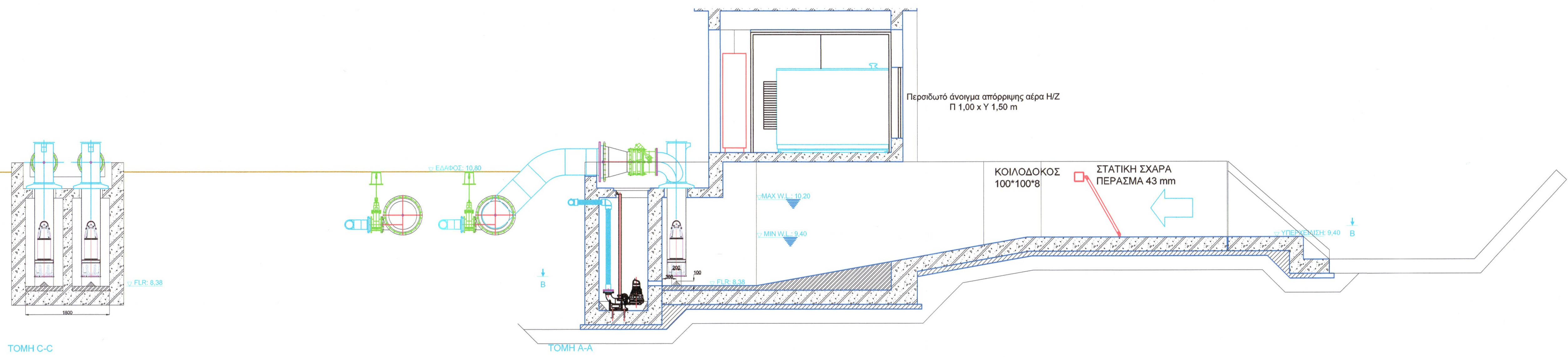
ΤΟΜΗ C-C
